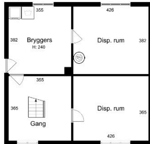
Kælder
