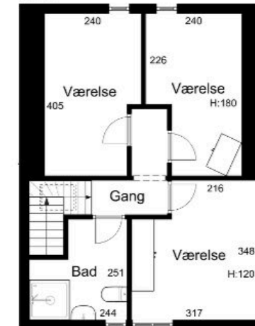
1. sal
