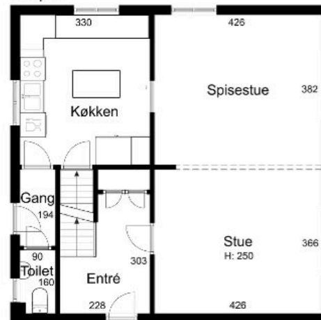
Stueplan
